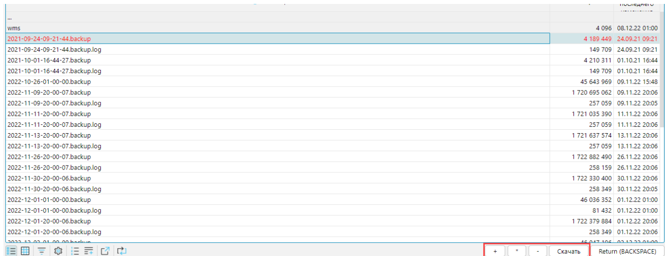
Рис. 2 Скачивание файлов
